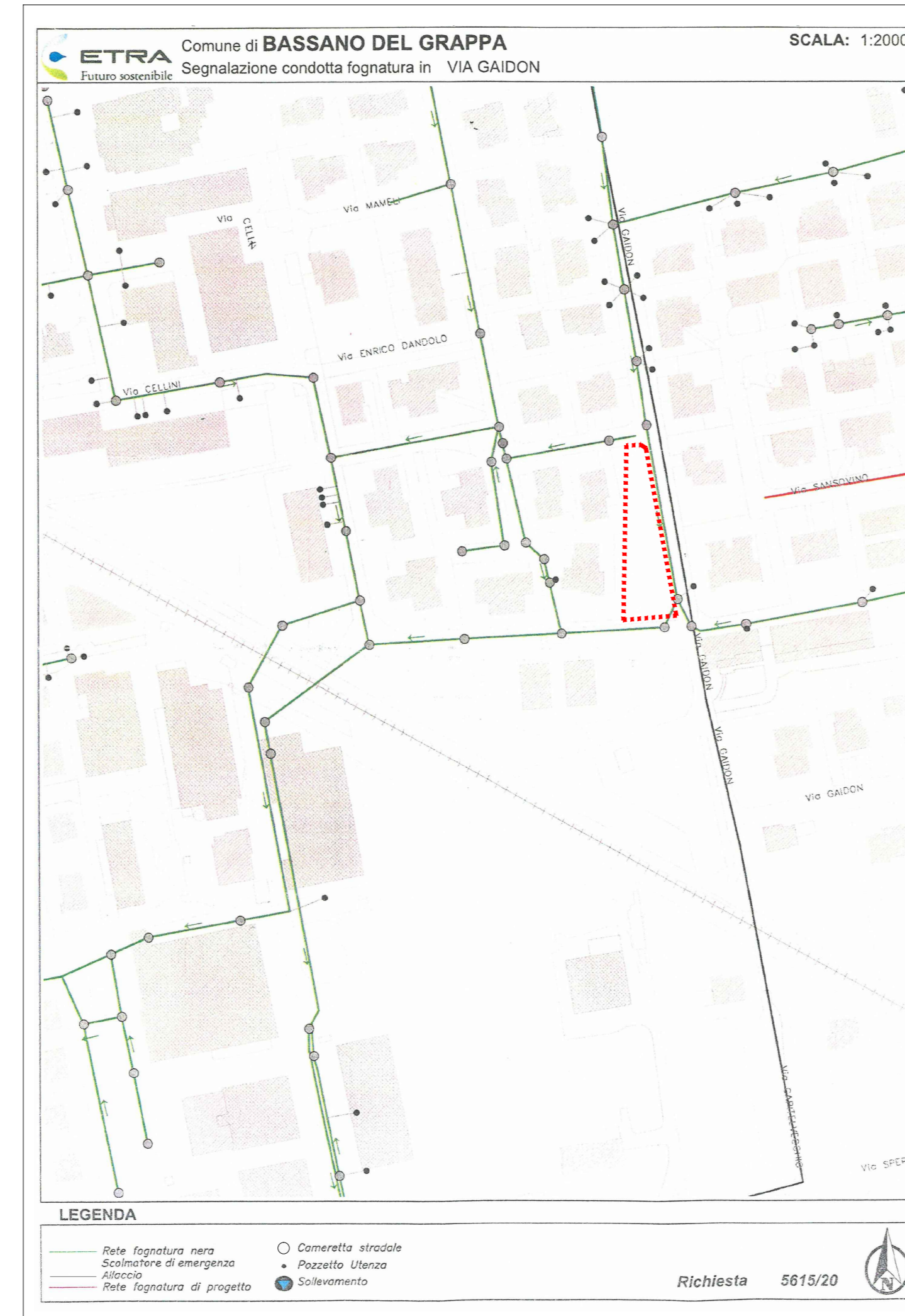
PLANIMETRIA DELLE INFRASTRUTTURE A RETE ESISTENTI CON IPOTESI DI ALLACCIAMENTO
